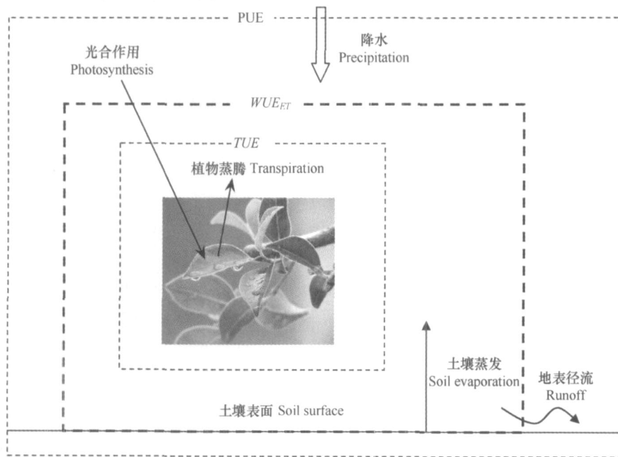
图 1 生态系统水分利用效率不同表达式所涉及过程示意图
