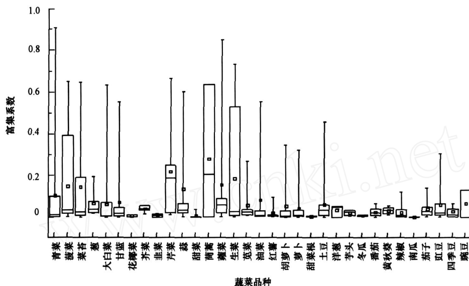
图 1 主要蔬菜品种的砷富集系数箱式图
