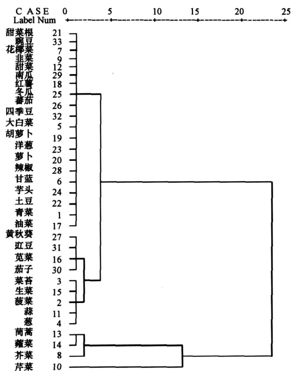
图 2 基于蔬菜砷富集系数几何均值的层级聚类分析结果
